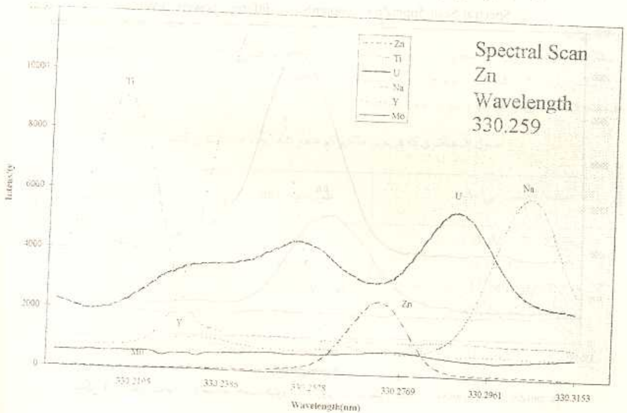
شکل ۴- اثر تغییرات در طول موج پلاسما بر روی شدت نشر عناصر Zn, Ti, U, Na, Y, Mo در طول موج ۳۳۰۲۵۹ نانومتر عنصر Zn
