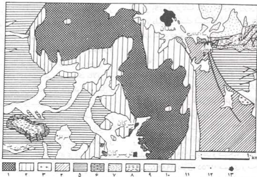
شکل ۱- نقشه زمین‌شناسی منطقه. ۱- نوده گرانیتوئید الوند، ۲- هورنلس و هورنلس‌سیت، ۳- پگماتیت، ۴- انواع سیت، ۵- اسلیت، ۶- آهک‌های ژوراسیک بالایی، ۷- ماسه‌سنگ کرتاسه، ۸- آهک و مارن کرتاسه، ۹- رسوبات میوسن، ۱۰- کواترنری، ۱۱- گل، ۱۲- روستا، ۱۳- شهر. (اقتباس با تغییراتی در چینه‌شناسی، از نقشه زمین‌شناسی
