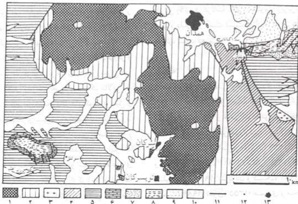
شکل ۱- نقشه زمین‌شناسی منطقه. ۱- نوده گرانیتوئید الوند، ۲- هورنلس و هورنلس‌سیت، ۳- بگماتیت، ۴- انواع سیت، ۵- اسلیت، ۶- آهک‌های ژوراسیک بالایی، ۷- ماسه‌سنگ کرتاسه، ۸- آهک و مارن کرتاسه، ۹- رسوبات میوسن، ۱۰- کواترنری، ۱۱- گل، ۱۲- روستا، ۱۳- شهر. (اقتباس با تغییراتی در چینه‌شناسی، از نقشه زمین‌شناسی
