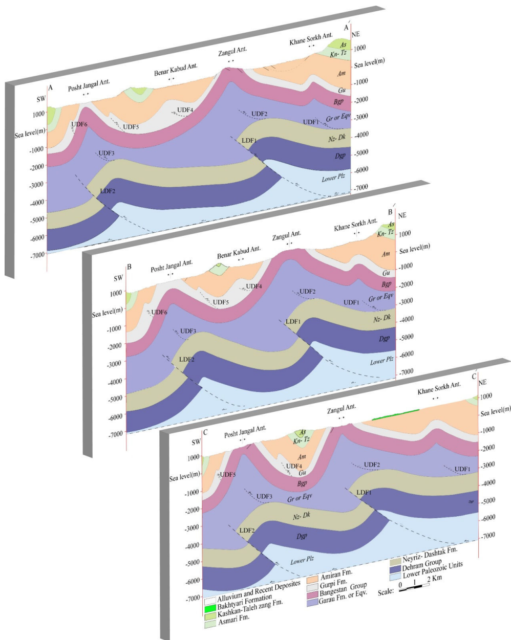
شکل ۹. تصویری از سه برش ساختاری تهیه شده بر روی تاقدیس زنگول
