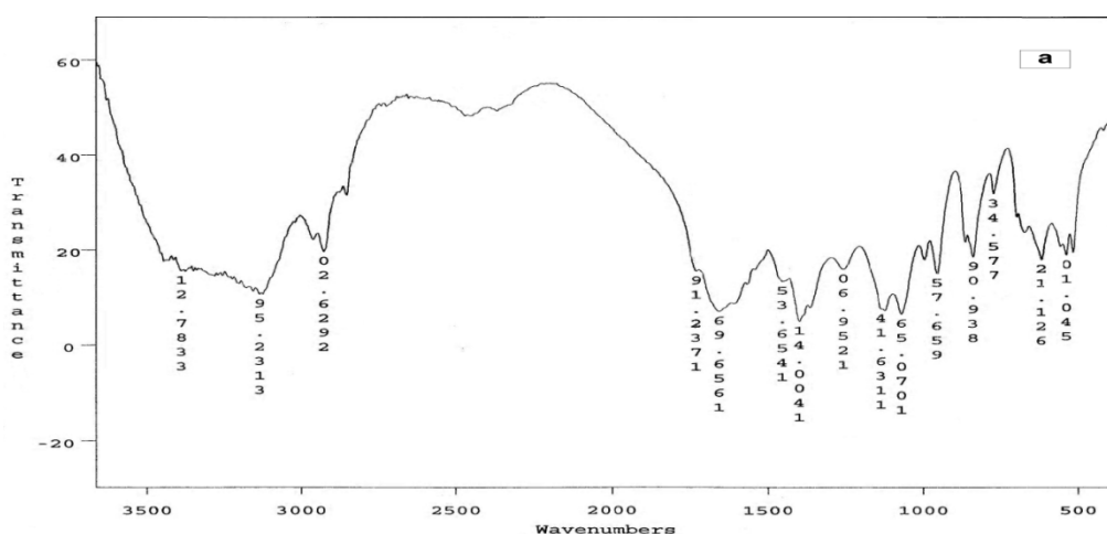
شکل ۳. الف) طیف FTIR سورفکتین تولید شده از باکتری باسیلوس سابیتیلیس NLIM ۰۱۱۰ تحت شرایط بهینه بیوراکتور (۳۷ °C و ۳۰۰ rpm و ۱/۵ vvm)
