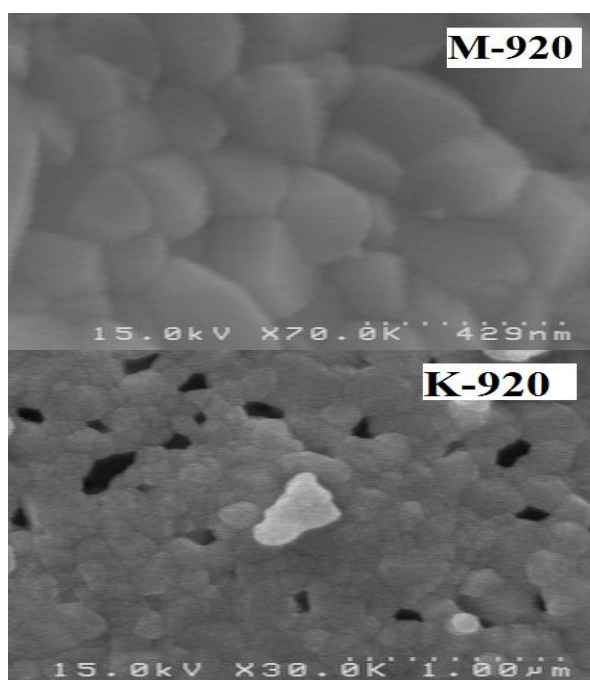
شکل ۵. تصاویر FE-SEM مربوط به نمونه‌های K-920 و M-920
