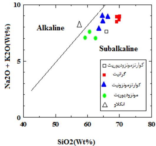
شکل ۱۱. نمودار تعیین سری ماگمایی [۱۶] برای تفکیک سری‌های ماگمایی آلكان و ساب آلكان در سنگ‌های منطقه بررسی شده
