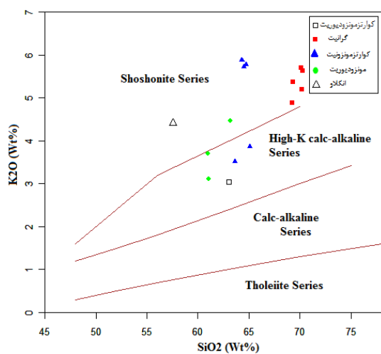
شکل ۱۰. نمودار آلكالی در برابر سیلیس [۱۵]
