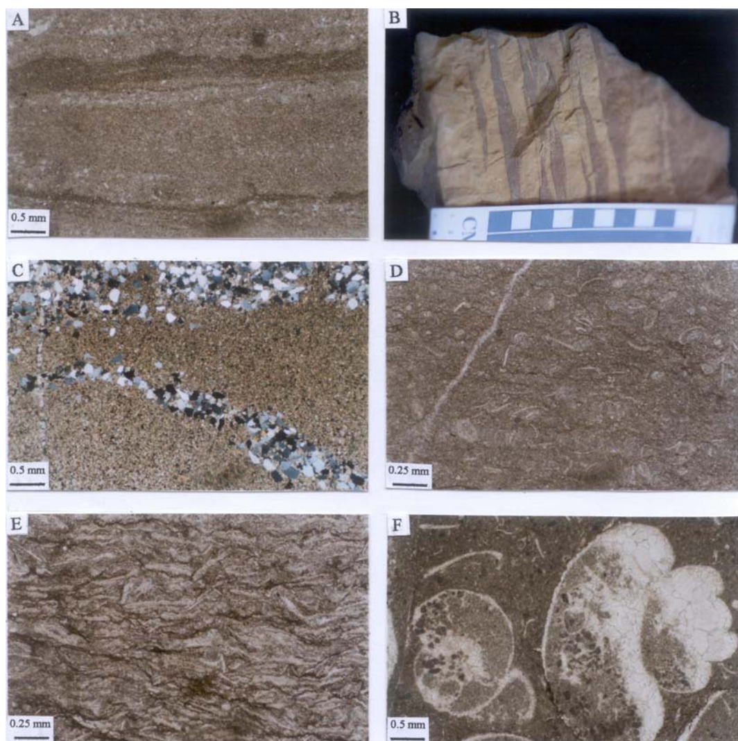
شکل ۳- A- بانداستون استروماتولیتی لامینه‌دار (زیر رخساره B4) در این تصویر، کلسیت اسپیری فابریک‌های چشم پرنده‌ای ریز را پر کرده است. (نمونه از برش گذار سرخ، نور طبیعی) B- نمونه دستی از دولومدستون با لایه‌بندی عدسی شکل (زیر رخساره B5) در این تصویر هر واحد از خطکش مقیاس برابر یک سانتی‌متر است. (نمونه از برش گذار گچال) C- تصویر بخشی از دولومدستون با لایه‌بندی عدسی شکل (زیر رخساره B5) لایه‌بندی‌های عدسی شکل از نظر سنگ‌شناسی، کوارتز آرنیت هستند. مقطع توسط آلیزاین قرمز رنگ‌آمیزی شده است. (نمونه از برش گذار گچال، نور پلاریزه) D- وکستون بیوکلاستی (زیر رخساره B6) بیوکلاست‌ها استراکندند (نمونه از برش گذار سرخ، نور طبیعی) E- پکستون بیوکلاستی (زیر رخساره B6) بیوکلاست‌ها شامل استراکندند (نمونه از برش گذار سرخ، نور طبیعی) F- تصویر دیگری از پکستون بیوکلاستی (زیر رخساره B6) بیوکلاست‌ها از شکم‌پایان (با برش‌های طولی، عرضی و فابریک ژنوپتال) هستند (نمونه از برش گذار گچال، نور طبیعی)
