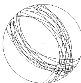
شکل ۸. الف) نمودار برگوارگی‌های نسل اول که دارای راستای شمال شمال باختر جنوب جنوب هستند ب) برگوارگی‌های نسل دوم در یک چین از نوع کینک در سنگ‌های سیلورین، خاور رشم. نگاه به جنوب باختر اندازه قلم داخل کادر: ۸ س.م
