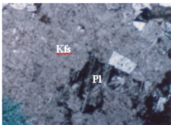
شکل ۵. تصویر بافت بوئی کلبیتی که در آن فلدسپات پتاسیک پلاژیوکلاز را در بر گرفته است ( \times 100.XPL ) فلدسپات پتاسیک = Kfs و پلاژیوکلاز = Pl
