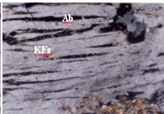
شکل ۸. نمایش بافت پرتیت (هم‌رشدی آلبیت و فلدسپات پتاسیک) در توده گرانیتی شمال موته ( \times 100.XPL ). فلدسپات پتاسیک = Kfs و آلبیت = Ab
