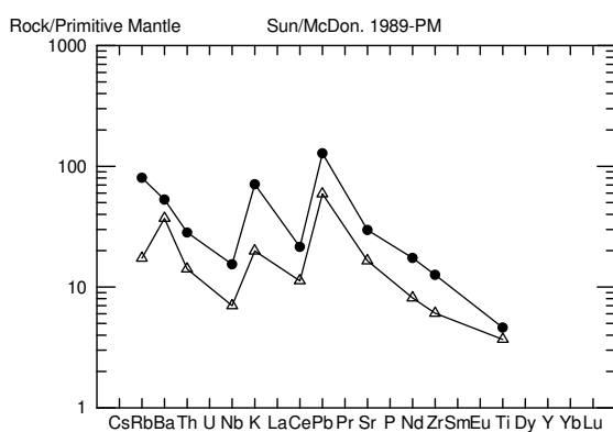
شکل ۹. مقایسه الگوی میانگین عناصر ناسازگار بازالت‌های جواهر دشت با مقادیر پوسته زیرین [۱۵] ● پوسته زیرین Δ بازالت‌های جواهر دشت
