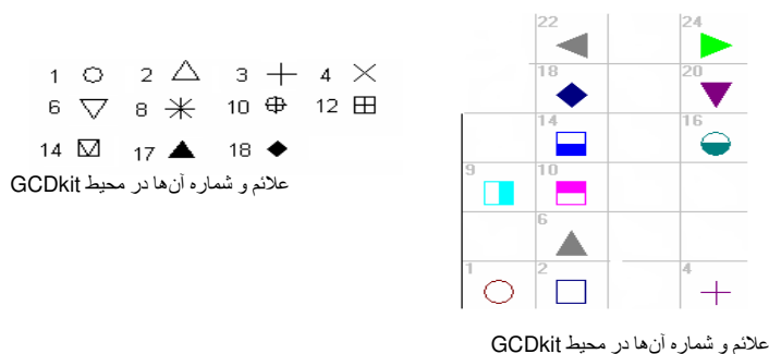
شکل ۳. در این شکل علائم و شماره آن‌ها در محیط‌های نرم افزاری GCDkit و minpet که در نمودارهای ژئوشیمیایی استفاده شده، نشان داده شده است
