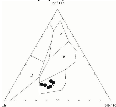
شکل ۱۱. نمودار متمایز کننده محیط تکتونیکی بر اساس عناصر غیرمتحرک. محدوده‌ها نماینده A: مورب نوع N، محدوده B: مورب نوع E و بازالت‌های تولیتی درون صفحه‌ای، محدوده C: بازالت‌های درون صفحه‌ای و محدوده D: بازالت‌های قوس آتشفشانی‌اند [۱۲]
