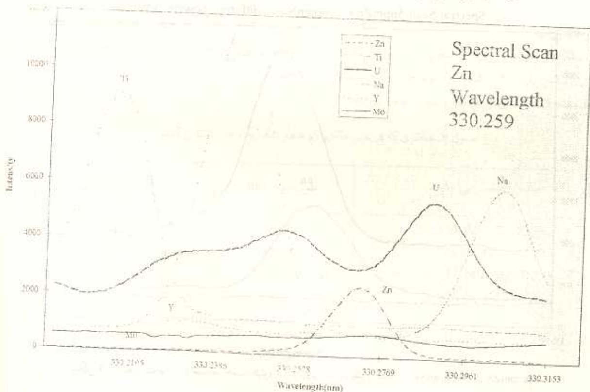
شکل ۴- اثر تغییرات در طول موج پلاسما بر روی شدت نشر عناصر Zn, Ti, U, Na, Y, Mo
