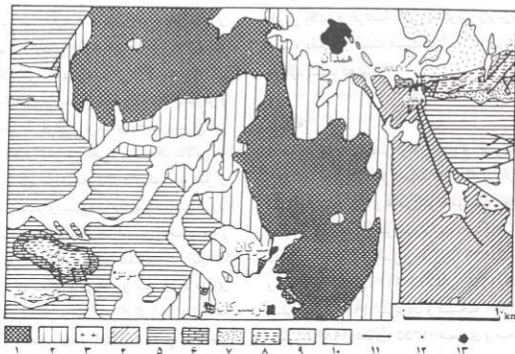
شکل ۱- نقشه زمین‌شناسی منطقه. ۱- نوده گرانیتوئید الوند، ۲- هورنلس و هورنلس‌شیت، ۳- بگماتیت، ۴- انواع شیت، ۵- اسلیت، ۶- آهک‌های ژوراسیک بالایی، ۷- ماسه‌سنگ کرتاسه، ۸- آهک و مارن کرتاسه، ۹- رسوبات میوسن، ۱۰- کواترنری، ۱۱- گل، ۱۲- روستا، ۱۳- شهر. (اقتباس با تغییراتی در چینه‌شناسی، از نقشه زمین‌شناسی
