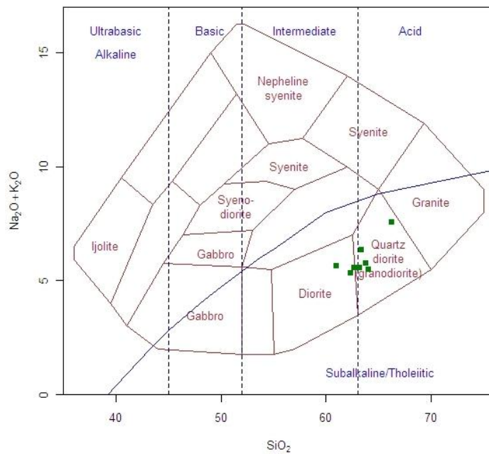
شکل ۲. موقعیت نمونه‌های بررسی شده در نمودار مجموع آلکان (TAS) در برابر SiO_2 [۱۷]. اغلب سنگ‌ها در محدوده ترکیبی کوچکی بین دیوریت و کوارتز دیوریت قرار گرفته‌اند
