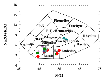
شکل ۳. طبقه‌بندی ژئوشیمیایی و نام‌گذاری سنگ‌های منطقه براساس مجموع آکالی در مقابل سیلیس (Cox et al., 1979)
