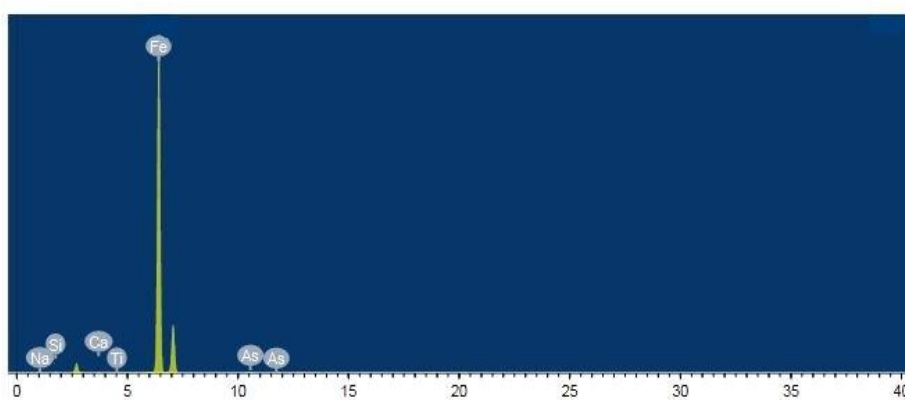
شکل ۵. طیف EDX نانوذرات \text{Fe}_3\text{O}_4
