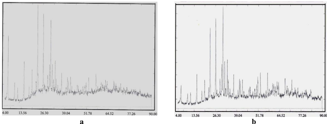
شکل ۴. الگوهای XRD (a) ۱۳X، (b) Nano-MnO 2 /Zeolite ۱۳
