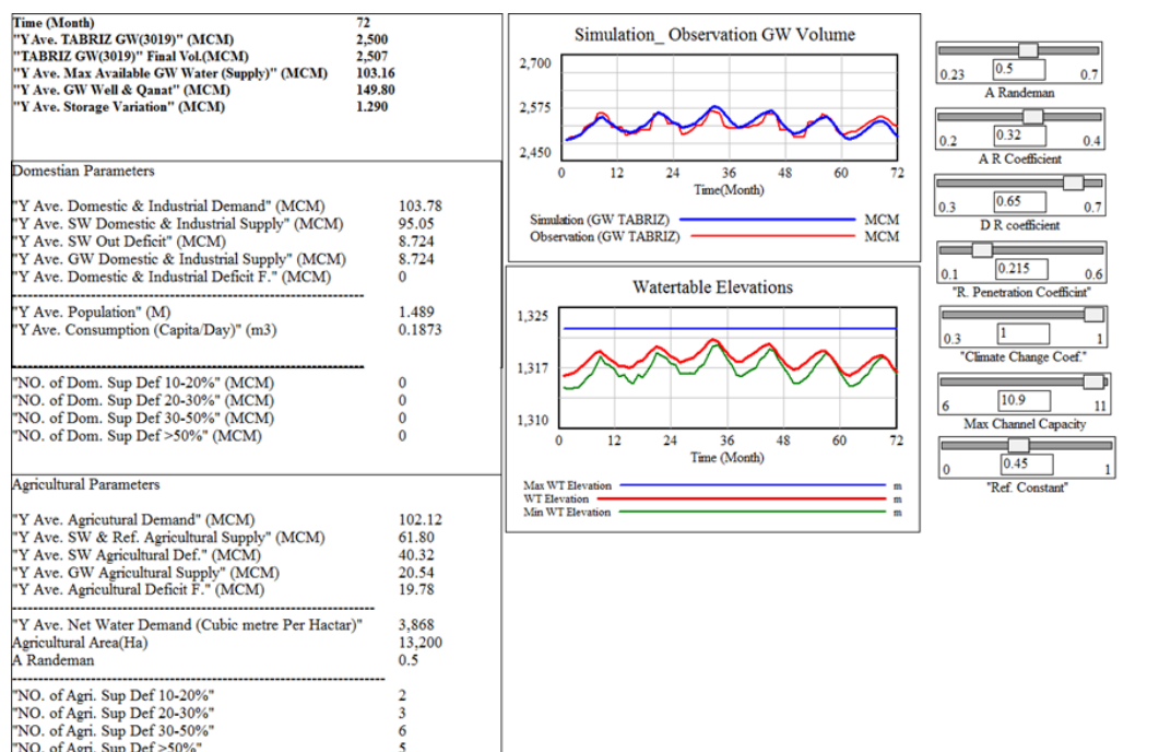
شکل ۱۱. سناریوی افزایش تخصیص از آب سطحی، افزایش بازده کشاورزی، توسعه شبکه جمع‌آوری فاضلاب و اجرای طرح تغذیه مصنوعی و اثرات حاصل از اجرای آن بر روی ذخیره آبخوان و پارامترهای نیاز کشاورزی
