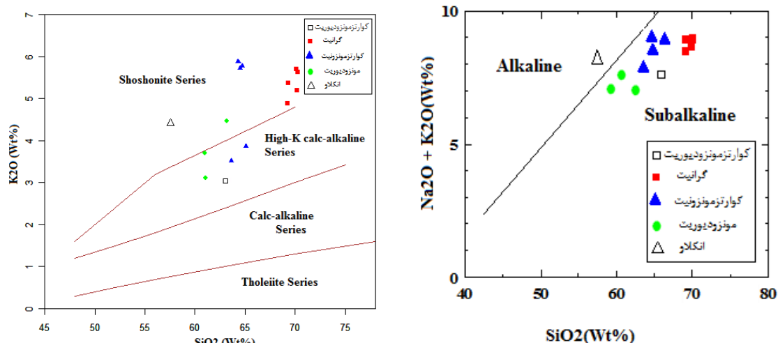
شکل ۱۰. نمودار آکالی در برابر سیلیس [۱۵]
