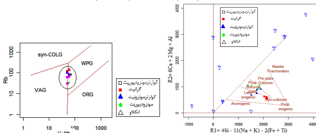
شکل ۱۸. نمودار تعیین محیط تکتونیکی توده‌های
