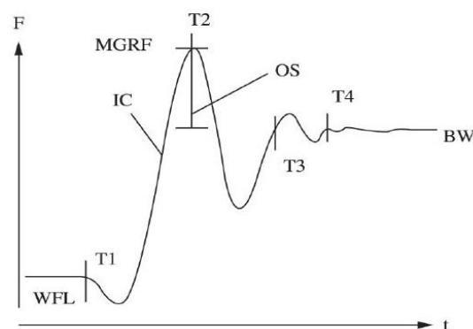
شکل ۱. نمودار مراحل حرکت نشست و برخاست به ۳ مرحله تقسیم‌بندی شده است. مرحله آماده‌سازی (T1-T2) مرحله برخاستن (T2-T3) مرحله ثبات (T3-T4) BW (وزن بدن)، MGRF (حداکثر نیروی واکنش زمین)، OS (میزان خطا)، IC (شیب)، WFL (وزن کف پا/پا) در استراحت، T1 (شروع حرکت)، T2 (نشسته)، T3 (برخاستن)، T4 (پایان حرکت) (۳۰)
