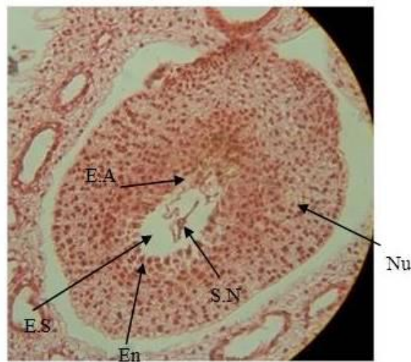
شکل ۱۴- برش عرضی تخمدان؛ Nu: خورش، E.A: دستگاه تخمزا، E.S: کیسه رویانی، En: اندوتلیوم، S.N: هسته ثانویه. بزرگنمایی 1920\times .
