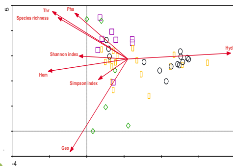
شکل ۳- تحلیل رسته‌بندی تطبیقی متعارف فاکتورهای آب مانداب بوجاق و کیشهر. گروه اول (○)، گروه دوم (◇)، گروه سوم (□)، گروه چهارم (▣).
