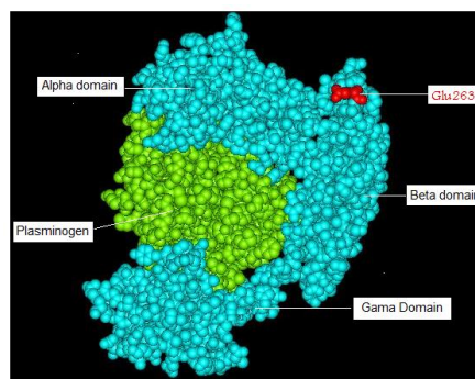
شکل ۲- ساختار کمپلکس استرپتوکیناز-پلازمینوژن. Fig. 2. Structure of streptokinase-plasminogen complex.
