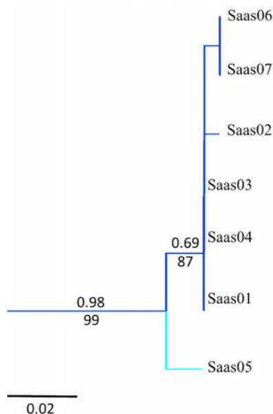
شکل ۲- درخت تبارشناختی گونه Saara asmussi . اعداد نمایش داده شده بر روی شاخه‌ها نشان‌دهنده Posterior probabilities بالای ۰/۵ در درخت BI (در بالای شاخه‌ها)، Bootstrap با ارزش بالای ۵۰ درصد برای درخت ML (در پایین شاخه‌ها) است. در اینجا ریشه‌ی درخت S. hardwickii نمایش داده نشده است.
