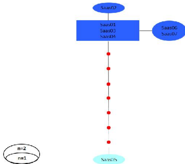
شکل ۳- شبکه آماری پارسیمونی بر اساس ژن میتوکندریایی سیتوکروم b، ارتباط درون گونه Saara asmussi در ایران را نشان می‌دهد. نقاط قرمز نشان‌دهنده هاپلوتایپ‌های از دست رفته یا نقاط نمونه برداری نشده است.
