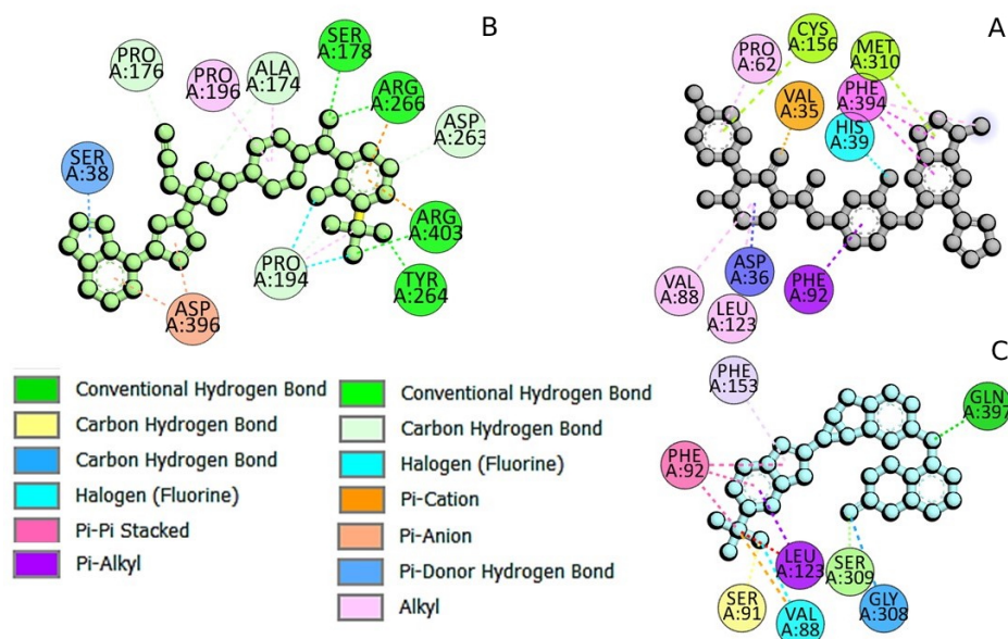
شکل ۱- برهمکنش آنزیم UGT1A1 با A) مرستینیب B) ایتاسیتینیب C) لیفرافنیب. ساختار لیگاندها در وسط هر تصویر و اسیدآمینه‌های آنزیم در اطراف آن نشان داده شده است. برهمکنش‌ها با نرم افزار دیسکاوری استودیو بررسی و تصویر آن ذخیره شد.
