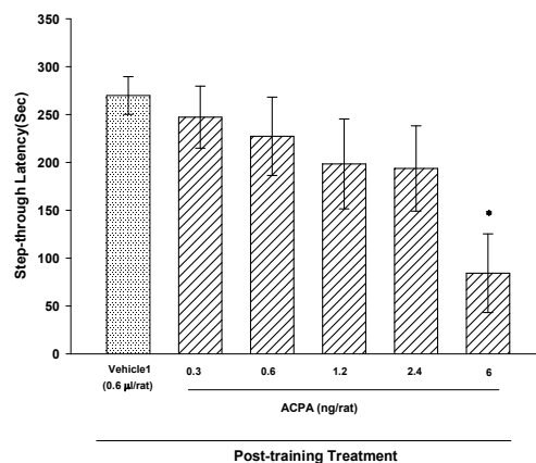
شکل ۱- مقایسه اثر تزریق ACPA به تنهایی با مقادیر مختلف (۰/۳، ۰/۶، ۱/۲، ۲/۴ و ۶ نانوگرم بر موش) بر حافظه اجتنابی مهاري نسبت به گروه کنترل (حامل ۱). داده‌ها بصورت میانگین (± خطای معیار) برای ۸ حیوان در هر گروه نشان داده شده است (* p<0.05 ).
