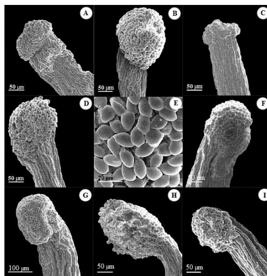
شکل ۱- تصاویر میکروسکوپ الکترونی نگاره از نمای کلی و سطح کلاله گونه‌های Pedicularis در ایران: (A) P. pycnantha (B) P. cabulica (C) P. wilhelmsiana (D) P. caucasica (E) نمایی از تزئینات سطح کلاله در گونه‌های Pedicularis به جز P. rhinanthoides (F) P. rechingeri (G) P. sibthorpii (H) P. rhinanthoides (I) P. condensata
