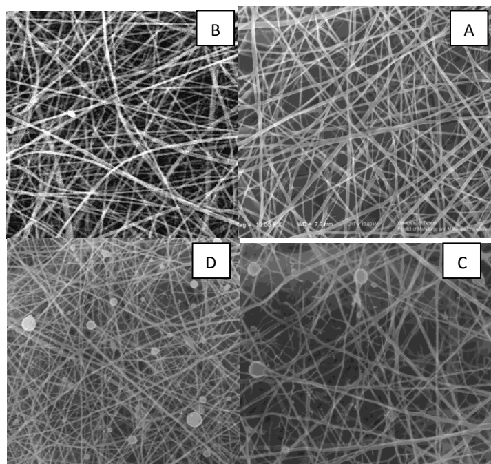
شکل ۱- تصویر میکروسکوپ الکترونی روبشی (SEM) نانوالیاف پلیمری الکترورسی شده. A: Chit/PEO 90:10، B: Chit/PEO/Li 1%، C: Chit/PEO/Li 2%، D: Chit/PEO/Li 3%.
