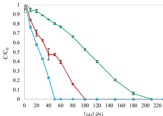
شکل ۱- تخریب PCA در دماهای مختلف (محلول در متانول، نگهداری شده در تاریکی)، ۲۵ درجه سانتیگراد (■)، ۳۵ درجه سانتیگراد (▲)، ۴۵ درجه سانتیگراد (●). Fig. 1. PCA destruction at various temperatures (PCA was kept in methanol in a dark bottle) 25°C (■), 35°C (▲), 45°C (●).
