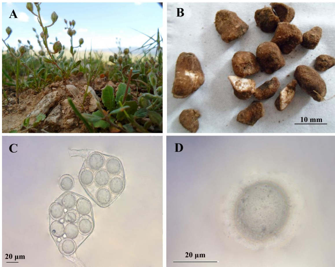
شکل ۲- ریخت‌شناسی گونه Picoa lefebvrei . A. گیاه میزبان ( Helianthemum ledifolium ). B. آسکوکارپ. C. آسک. D. آسکوسپور.
