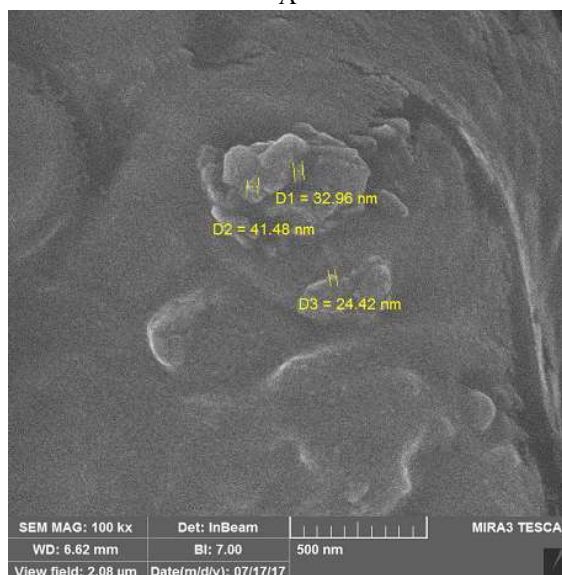
شکل ۶- تصاویر SEM از تجمعات کریستالها تولید شده توسط جدایه ۶ بر روی سطوح باکتری در محیط رسوبی با بزرگنمایی‌های مختلف. A . 5kx. B . 100kx. Fig. 6. SEM images of aggregation of nanocrystals produced by isolate 6 on bacterial cell surfaces in precipitating medium with different magnifications. A . 5kx. B . 100kx.
