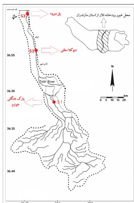
شکل ۱- نقشه حوضه آبریز رودخانه تالار و ایستگاه‌های نمونه‌برداری
