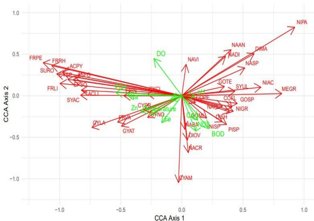
شکل ۲- رسته‌بندی CCA گونه‌های‌های اپی‌لیتیک دیاتومه‌ها براساس متغیرهای محیطی
