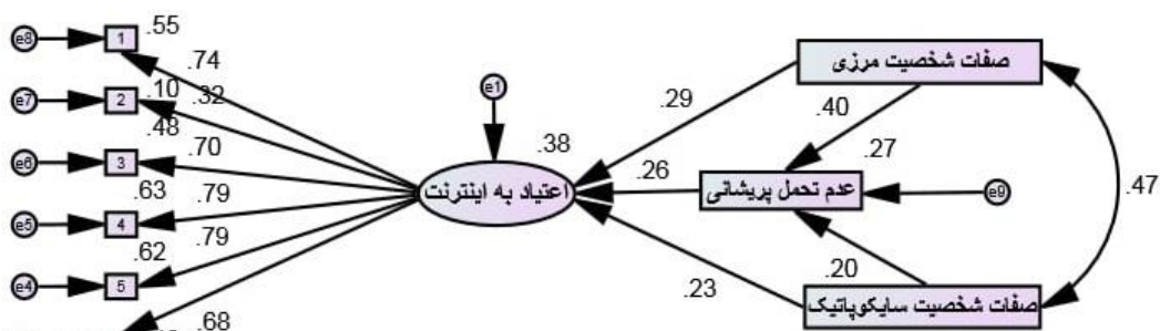
شکل ۲. تحلیل مسیر اعتیاد به اینترنت بر اساس صفات شخصیتی مرزی و جامعه‌ستیزی به واسطه نقش میانجی عدم تحمل پریشانی
