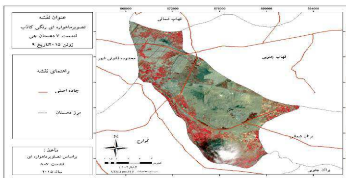
شکل شماره (۵): تصویر ماهواره‌ای رنگی کاذب هندست ۷ دهستان جی، تاریخ ۹ ژوئن ۲۰۱۵ منبع: تصاویر ماهواره‌ای هندست ۷ و ۸
