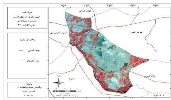
شکل شماره (۴): تصویر ماهواره‌ای رنگی کاذب هندست ۷ دهستان جی، تاریخ ۷ ژوئن ۲۰۰۸
