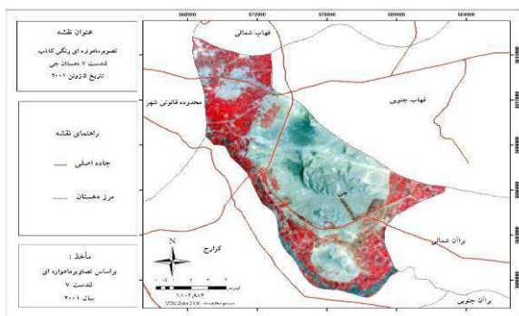
شکل شماره (۳): تصویر ماهواره‌ای رنگی کاذب هندست ۷ دهستان جی، تاریخ ۵ ژوئن ۲۰۰۱
