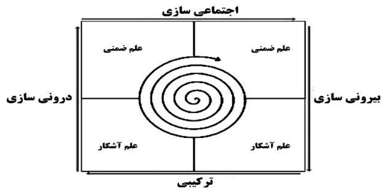
شکل ۱. مدل SECI
